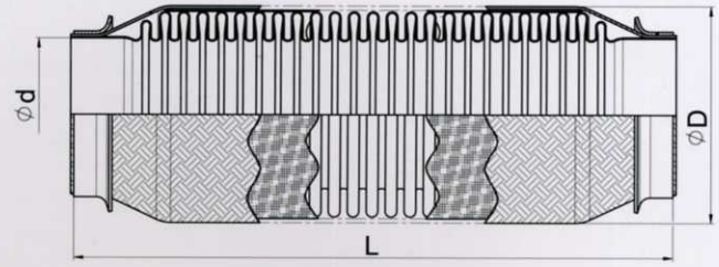
İÇ ÖRGÜSÜZ / WITHOUT INNER BRAID
