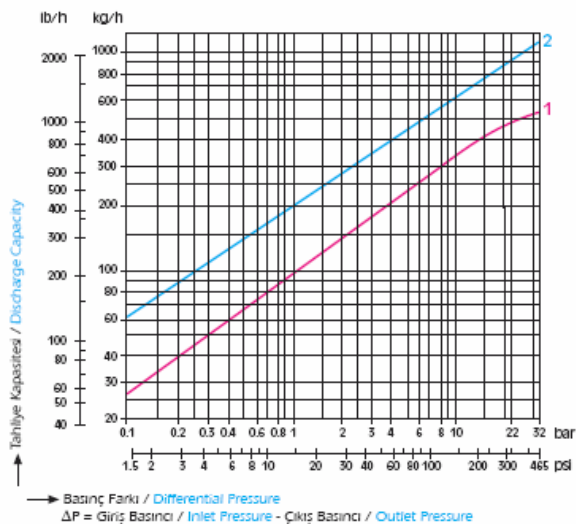
Tahliye Miktarları / Discharge Capacities ( 3/8" - 3/4" )
