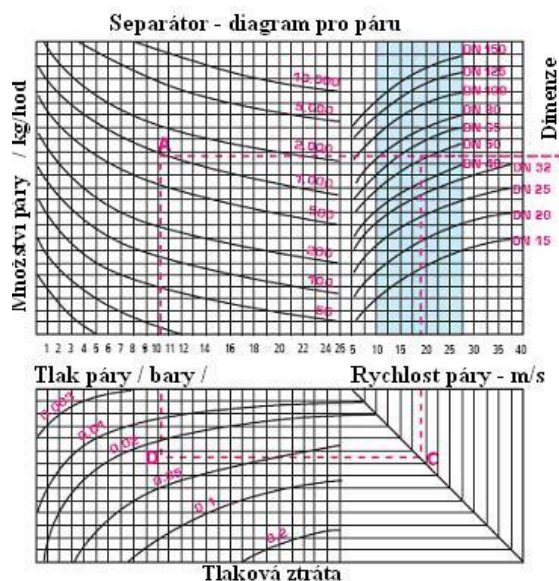
ROZMĚRY SEPARÁTORU
