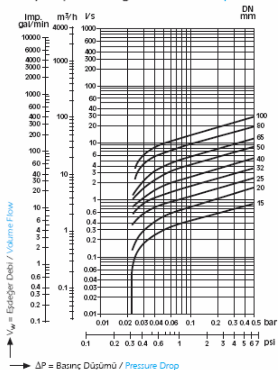
Basiç Düşüm Grafiği / Pressure Drop Chart
